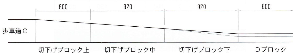
切下げ部施工図
