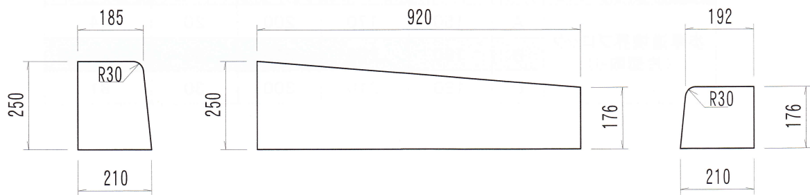
切下げブロック中 参考重量/88kg
