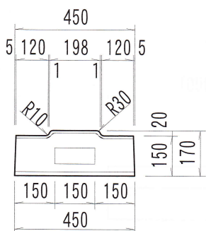
平 20 参考重量/321kg
