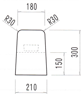
水抜 参考重量/60kg
