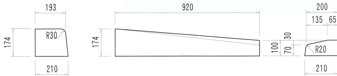
切下げブロック下 参考重量/56kg
