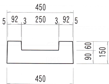
基礎ブロック L=600 参考重量/72kg L=900 108kg
