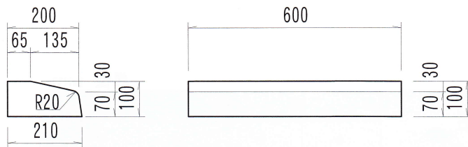
切下げ部施工図
