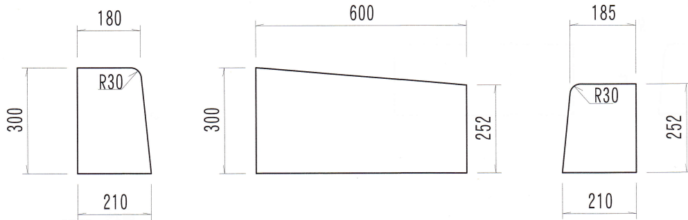
切下げブロック上 参考重量/75kg
